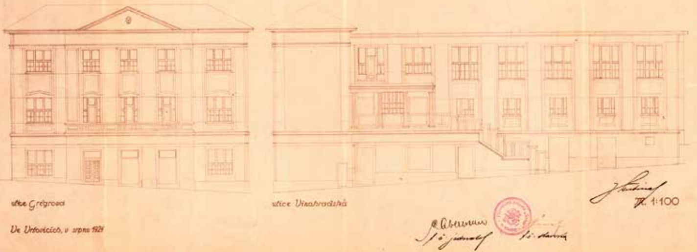
NÁVRH FASÁDY VZLETU OD JOSEFA KUTINY
