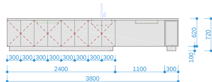
pohled od tabule směrem do učebny
