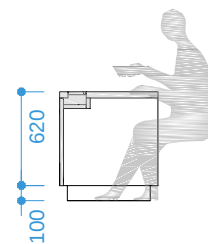
příčný řez v místě katedry
